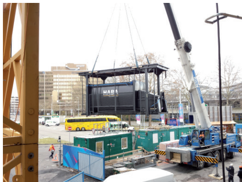
HABA MEGA järjestelmän asennus valmiiseen kaivantoon kestää 3-4 tuntia.
